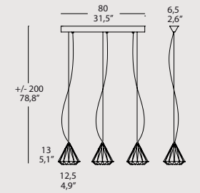
KARAT S3L 3 x MAX 42W G9 alo. ENERGY SAVER CE F IP 20 1 ENEC
