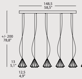
KARAT SSL 5 x MAX 42W G9 alo. ENERGY SAVER CE F IP 20 1 ENEC
