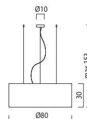
Sospensione - Pendant S2 4x24W E27 TC-TSE 4x12W CLASSIC A LED (E27) CE E IP 20
