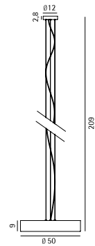
Sospensione - Pendant CE VF IP 20
