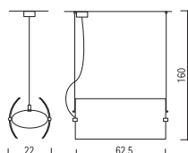
Sospensione - Pendant L62 CE
