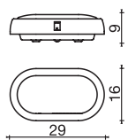
Parete/soffitto - Wall/ceiling P1
