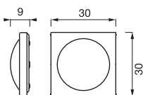
Parete/soffitto - Wall/ceiling A4 CE IP 30
