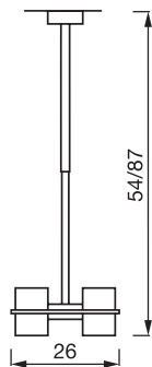
Sospensione - Pendant S CE IP30
