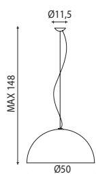
Sospensione - Pendant S2
