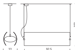
Sospensione - Pendant L92 CE
